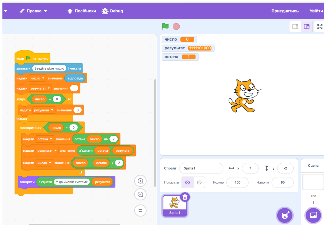
Рис. 1 Двійкова система.
