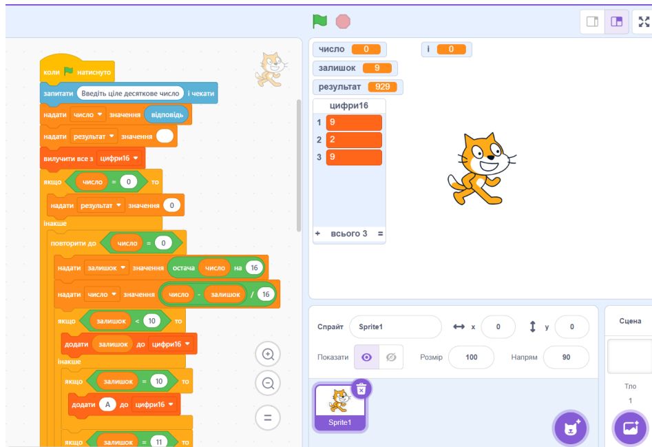
Рис. 2 Шістнадцяткова система.
